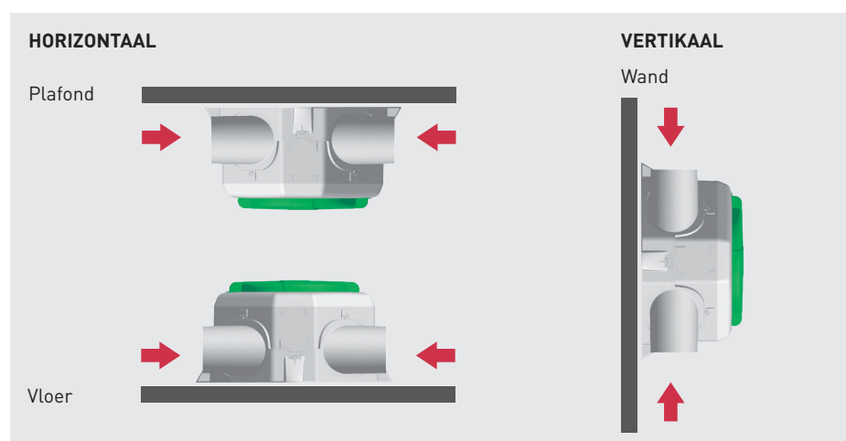
Montage voorbeeld
