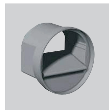
RD BP Speciale automatisch geregelde lagedruk-volumeregelaar (20-100 Pa) met mof voor directe montage in het kanaal. Diameter 80 mm. Luchtdebiet: 15 of 30 m³/h.
