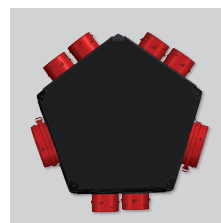
PLENUM UNI EXT 6+1 Geïsoleerd afzuigplenum met een diameter van 125/150-160 mm, 1 aansluiting met een diameter van 125 mm voor de keuken en max. 6 aansluitingen met een diameter van 80 mm voor sanitaire voorzieningen.
